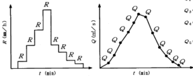
タイムエリア法による有効降雨・流出ハイドログラフ
