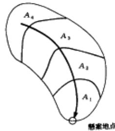
タイムエリア法による到達時間域図
