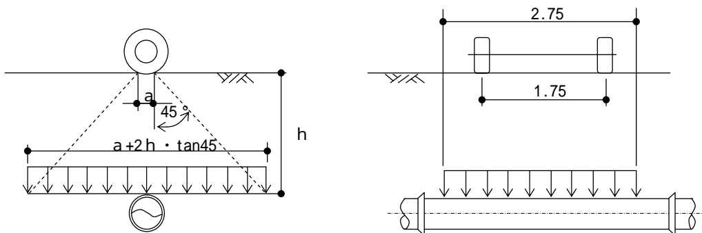
図-2自動車荷重の分布図
